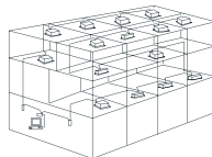
Схема подключения с надежной связью
