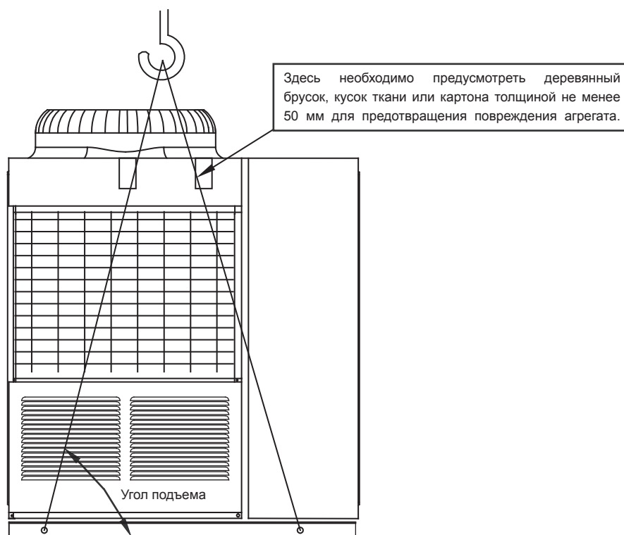
Рис. 2-1 Подъем агрегата
