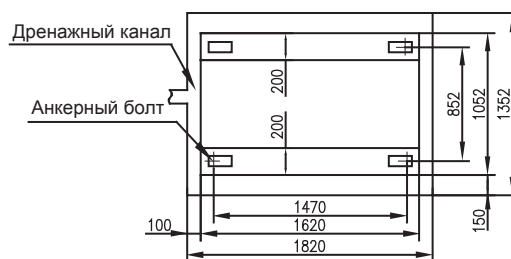
Схема с установочными размерами агрегата
